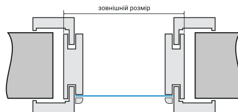
Конструкція фрамуги у виконанні VERTO-FIT
