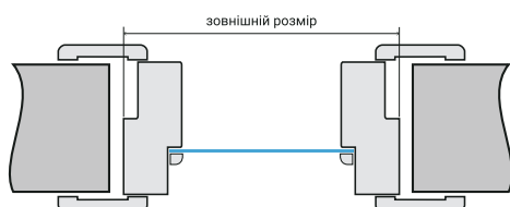
Конструкція фрамуги у виконанні STANDARD
