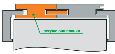
Переріз дверної коробки із регулюючою планкою та шпонкою
