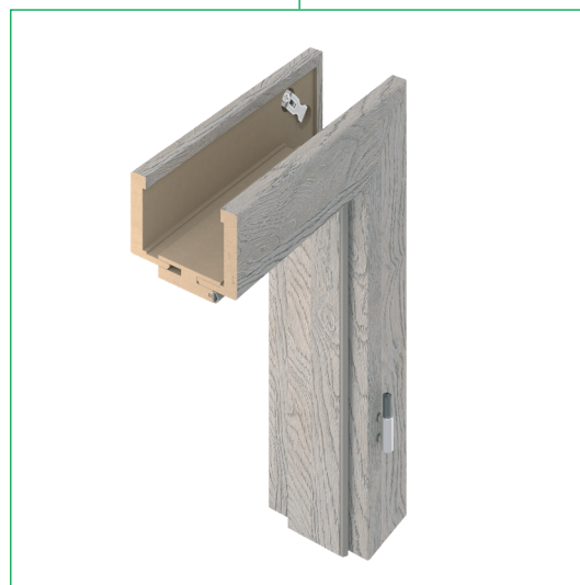
Переріз дверної коробки із регулюючою планкою та шпонкою
